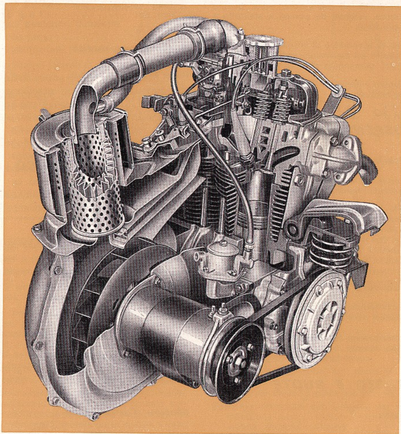
Motore con ventilatore, sezionati parzialmente
